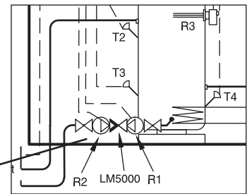
Fig. 7 Vid inkoppling och användning av Sys 31 placeras lämpligen pumpar och givare enligt ovan.
